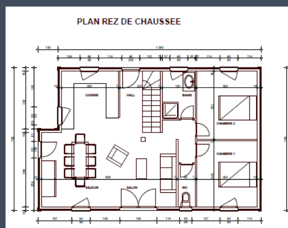
Plans de la maison Urbana grand modèle, combles aménagés
